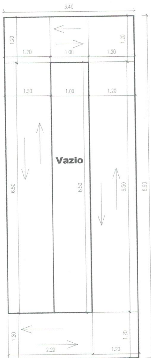
PLANTA BAIXA Esc.: 1/75 Á: 25,20m 2
